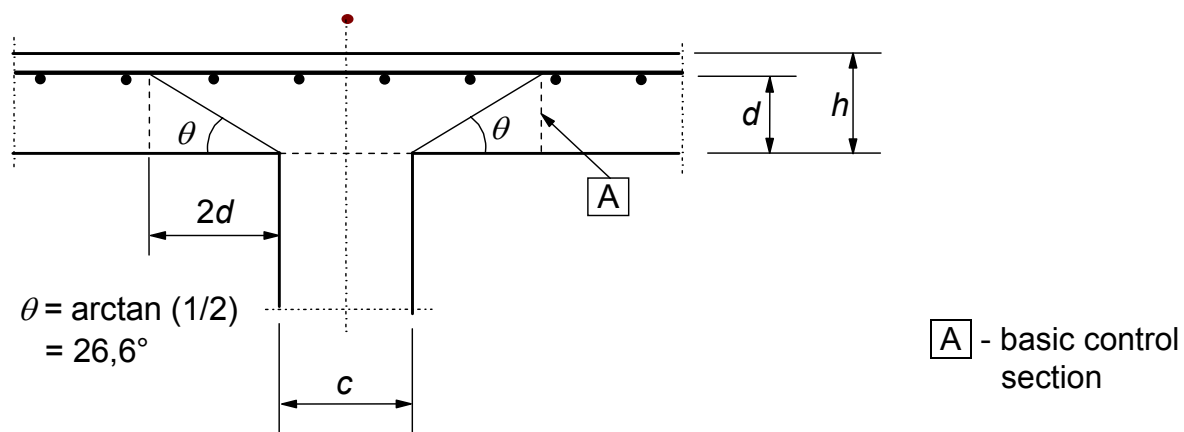
a) Section
