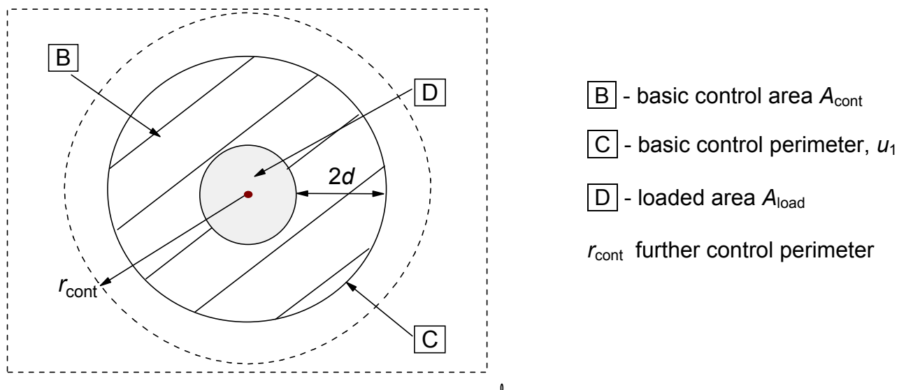
b) Plan
