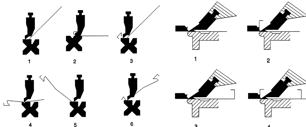
Press braking
